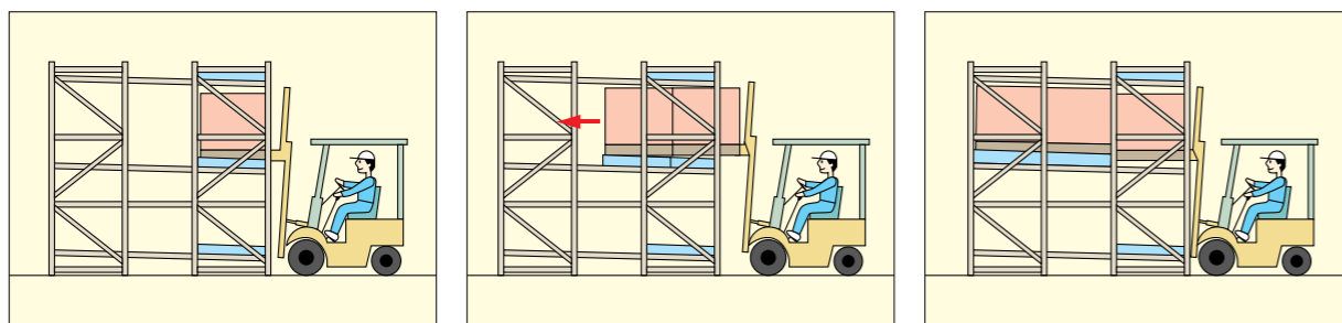
A 収納物を台車に載せます。 B 最初の収納物を押し込みながら次の台車に収納物を載せます。 C 収納物を押し込みながら最後はレールの上に収納物を載せます。
