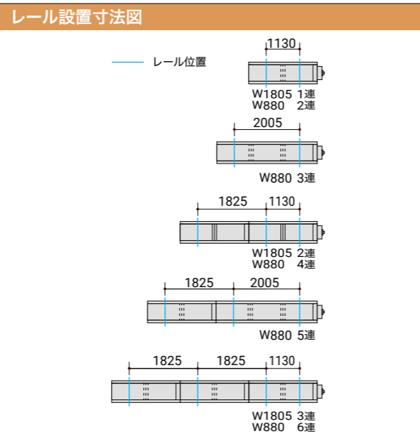
※レール設置寸法は、レール中心線を基準としています。
