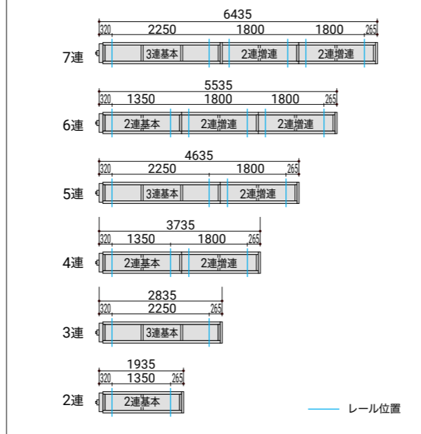
レール設置寸法図
